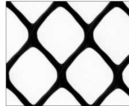
呼称 HX25A 網目の大きさ(ピッチ) : a19mm x b19mm サイズ(幅 x 長さ) : 124cmx30m 色 : 黒 | 主材料 : 高密度ポリエチレン
