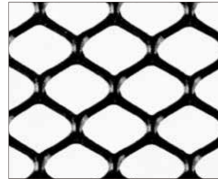
呼称 D7 網目の大きさ(ピッチ) : a12mm x b12mm サイズ(幅 x 長さ) : 91cmx30m 色 : 黒 | 主材料 : 高密度ポリエチレン
