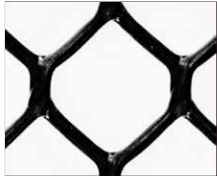
呼称 WF1 網目の大きさ(ピッチ) : a27mm x b27mm サイズ(幅 x 長さ) : 62cmx30m, 124cmx30m, 200cmx30m 色 : 黒 | 主材料 : 高密度ポリエチレン
