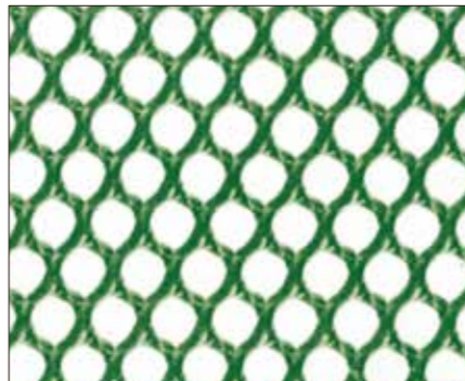
呼称 AN3 網目の大きさ(ピッチ) : a5mm x b5mm サイズ(幅 x 長さ) : 30cmx30m, 40cmx30m, 62cmx30m, 124cmx30m 色 : 濃緑 | 主材料 : 高密度ポリエチレン
