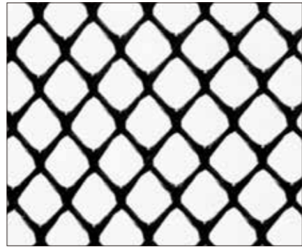
呼称 WF4 網目の大きさ(ピッチ) : a8mm x b8mm サイズ(幅 x 長さ) : 124cmx30m 色 : 黒 | 主材料 : 高密度ポリエチレン
