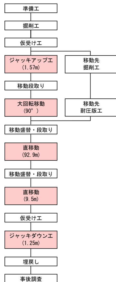
施工フロー
